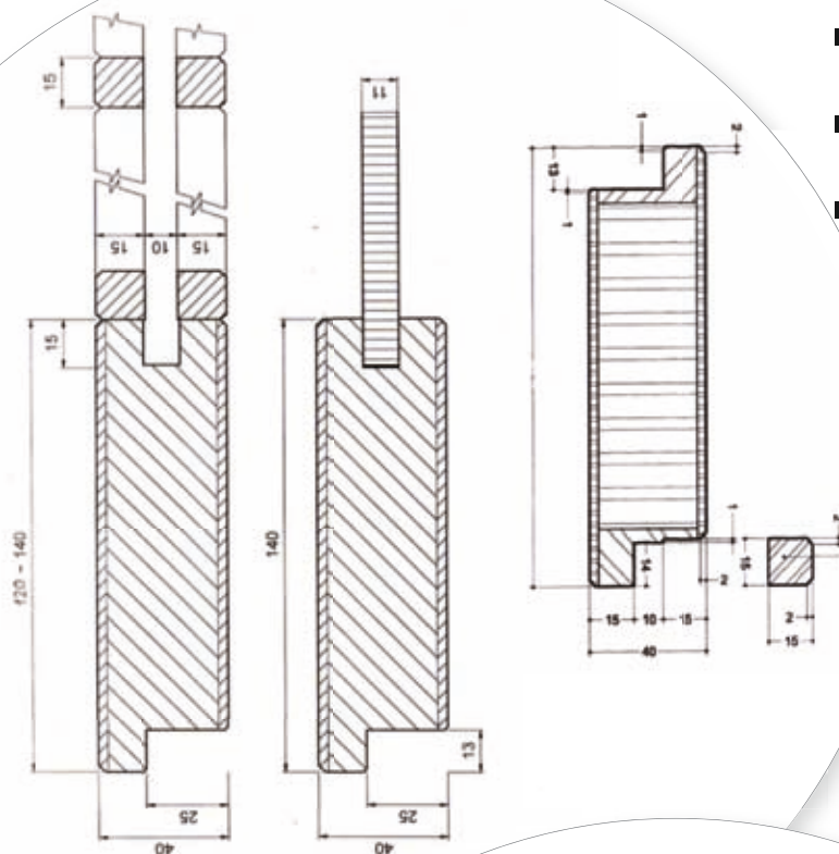
kulatá profilace FG pro řadu FG a G
